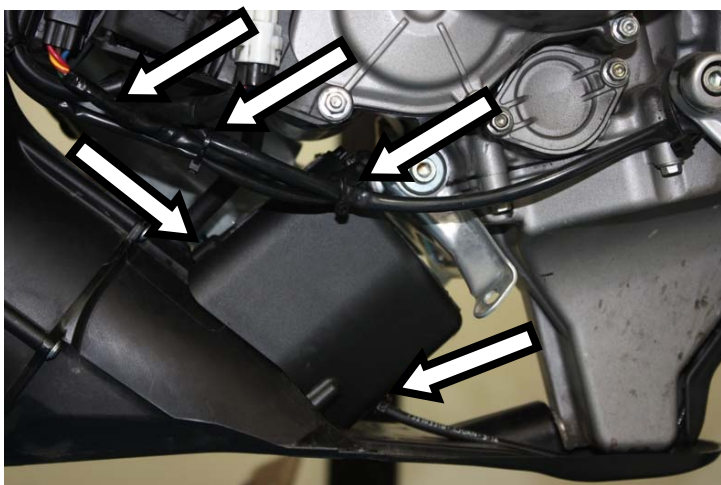
Tagliare le fascette a strappo di tutti i cablaggi posti in prossimità del coperchio motore attuatore valvola Cut and remove all the straps securing the exhaust valve cables near the cover of the actuator engine
