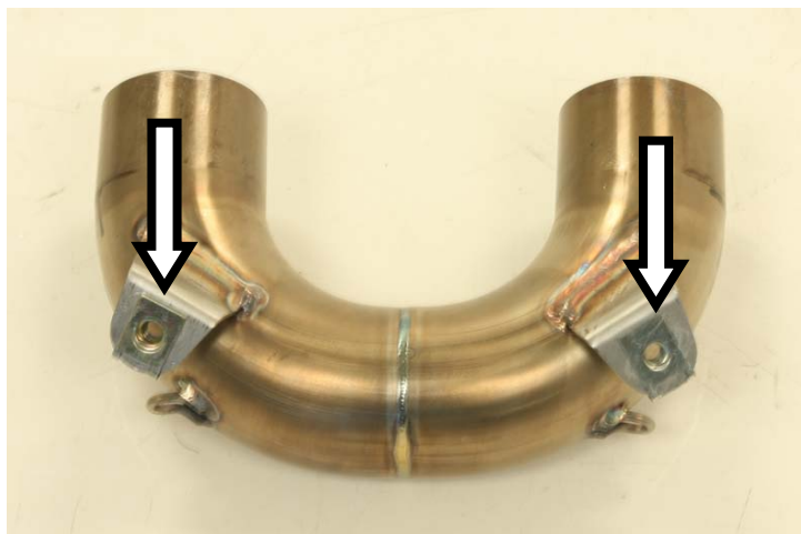
Inserire negli attacchi del raccordo le clip M6 Fit M6 caged nuts to the mounting points in the link pipe
