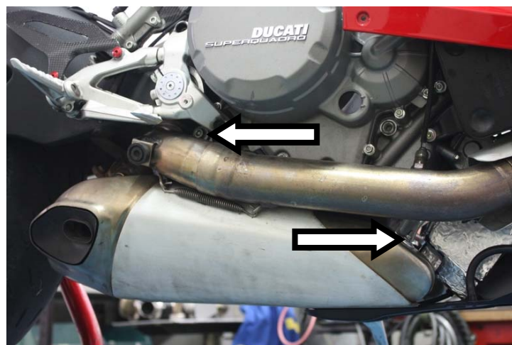
Svitare le viti di fissaggio (2 per lato) e rimuovere lo scarico Unscrew the screws (2 on each side) and remove OE silencers
