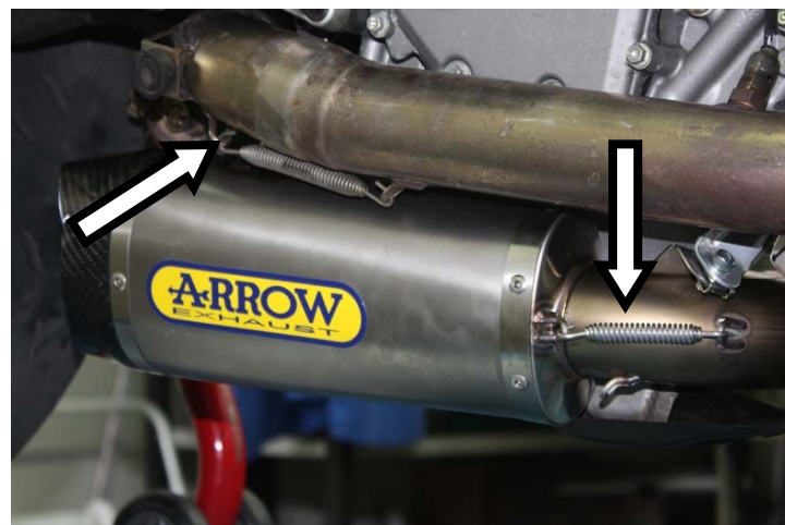
Ripetere l'operazione per il terminale DX e rimontare le carene. Repeat the same operations for the RH silencer. Fit the bodywork in its place
